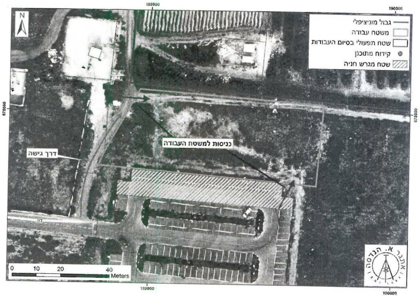
איור 1. משטח העבודה של הקידוח, מיקום משוער של הקידוח והשטח התפעולי בסיום העבודות
